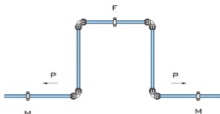
Expansielus, gebruik gemaakt van vier 90° bochten
